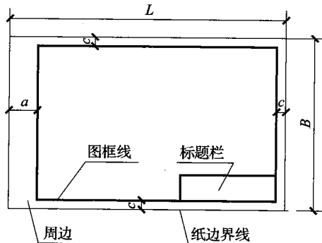
图 3.1.7 图框格式
